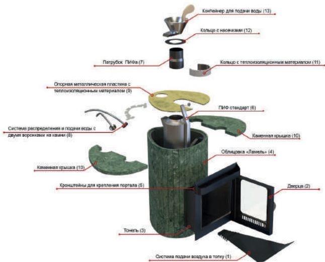
Рис. № 11 Схема установки ПИФ на печь
